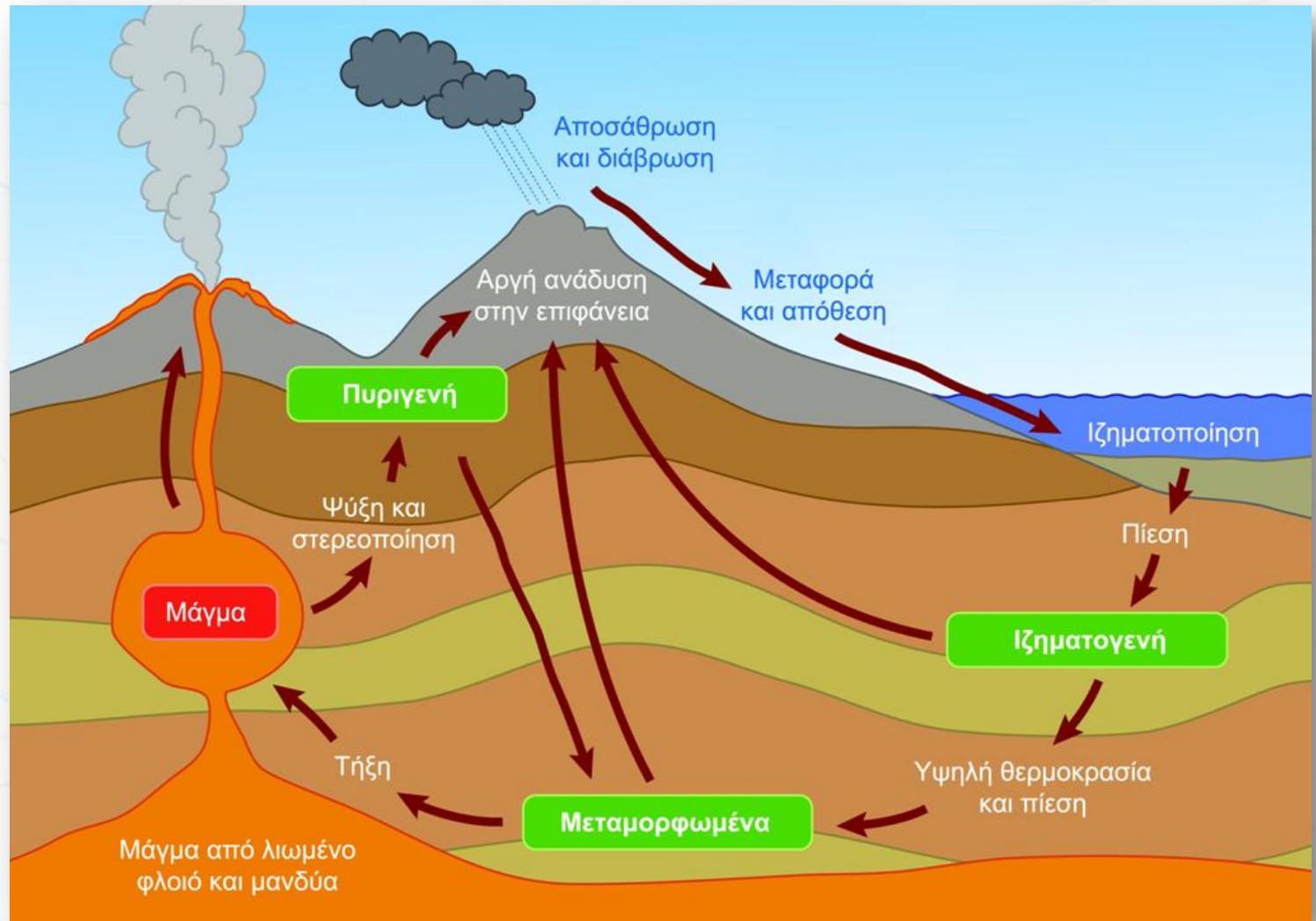
Εικόνα 3. Πετρολογικός κύκλος
